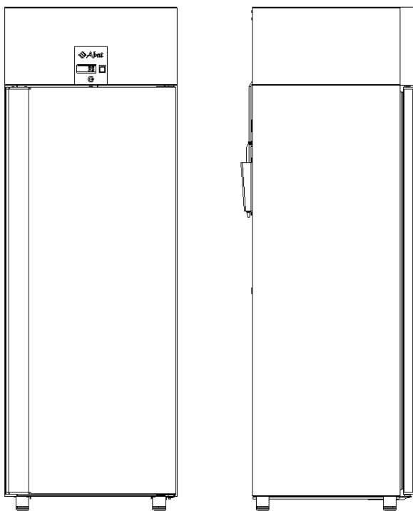
Рис. 2. ШХс-0,5Т; ШХс-0,5Т-01; ШХс-0,7Т; ШХс-0,7Т-01 с верхним расположением АКК
